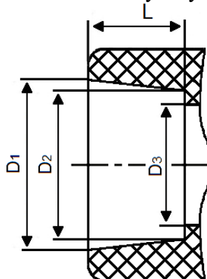
Рис 2. Раструбная часть фитингов
