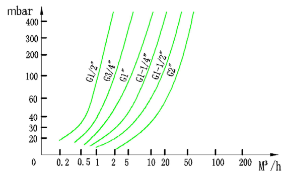
График зависимости потерь давления от расхода
