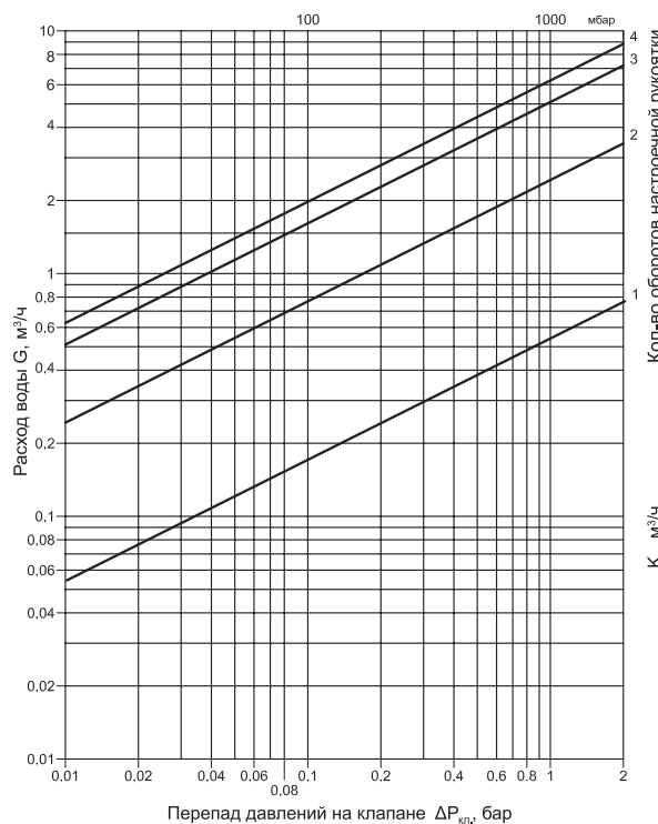
Диаграмма для настройки клапана MNF DN = 20 мм
