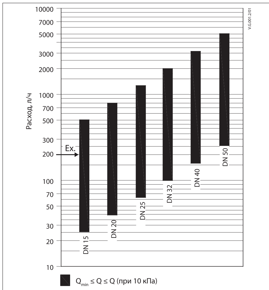
Диаграмма подбора клапана АРТ при \Delta P_{бк} = 10 кПа
