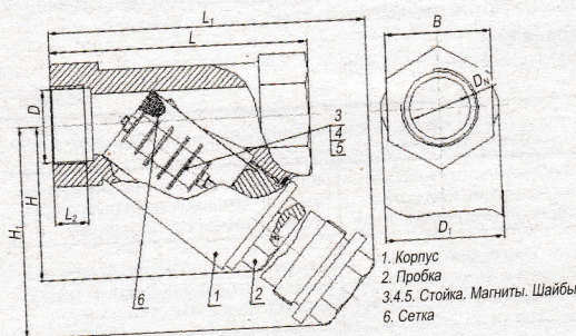
Конструкция фильтра ФСМ, ФС исп. 1
